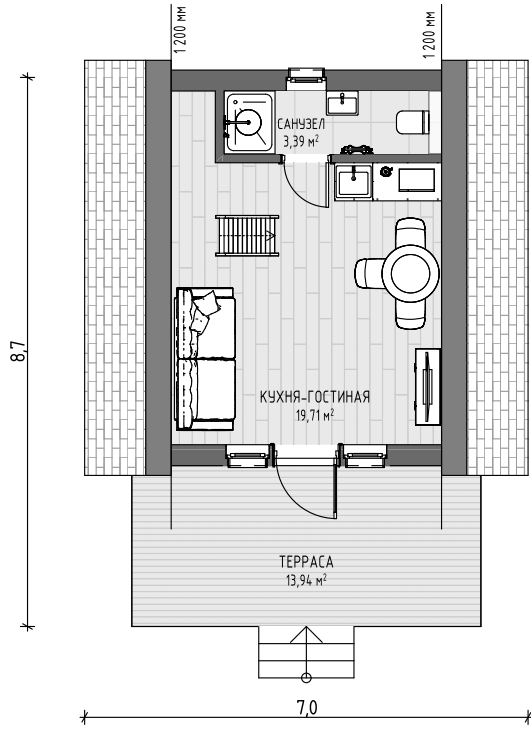
Планировка 1-го этажа
